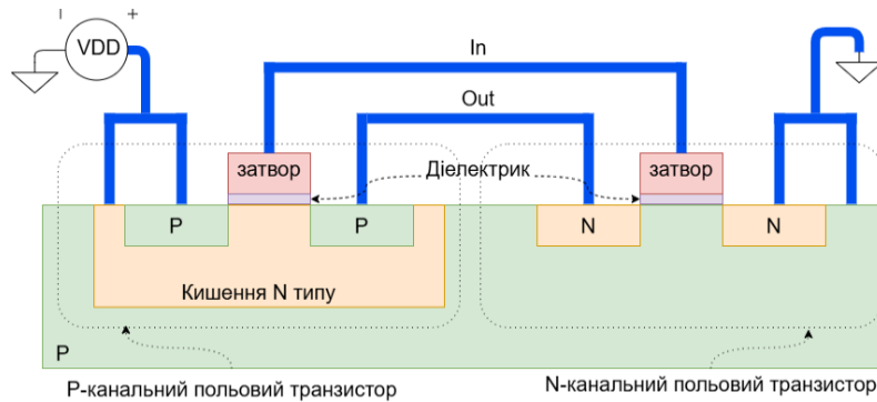
Рис. 1. КМОН інвертор на підкладці р-типу
